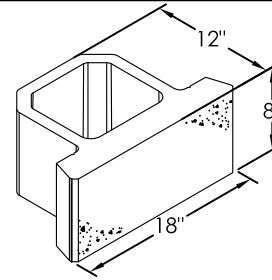
Premier 8 unit (Straight Split)
